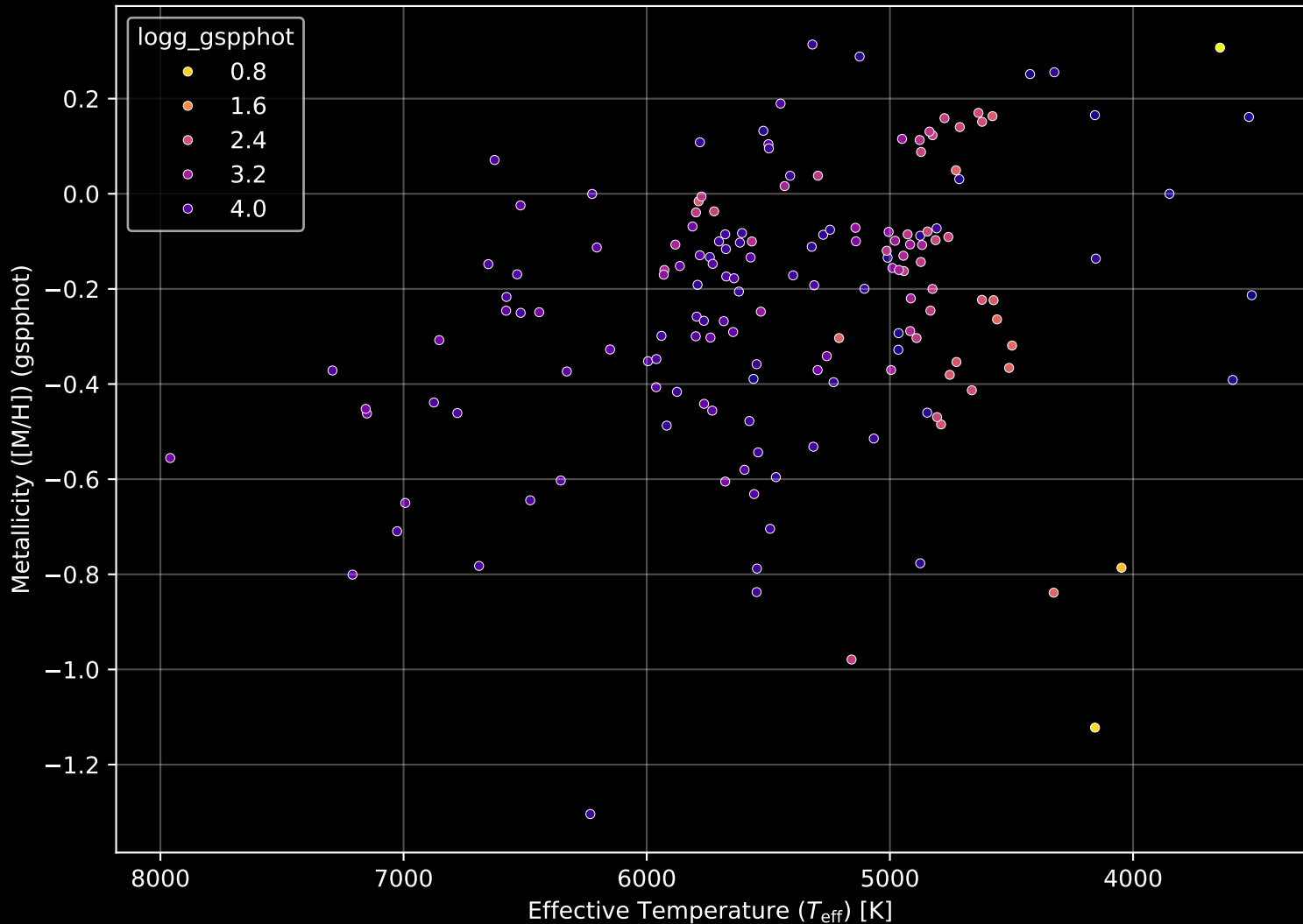
APOGEE DR17 Field: [065-29_MGA] Stellar Population Parameters (n= 161)
